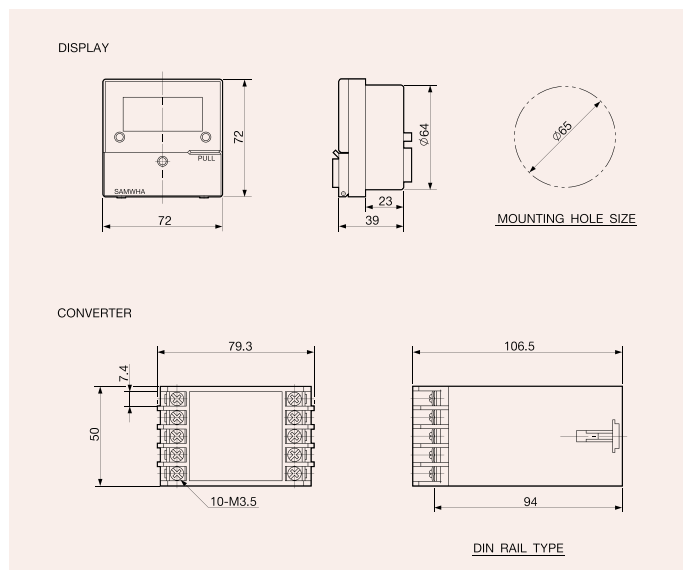
EVR-FD
