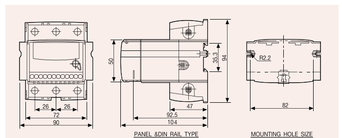
EOCR-PMZ
