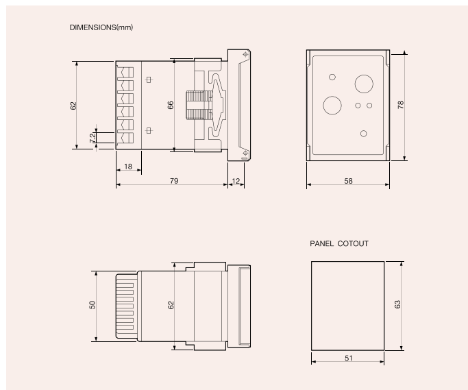
ELR / EFR2.5
