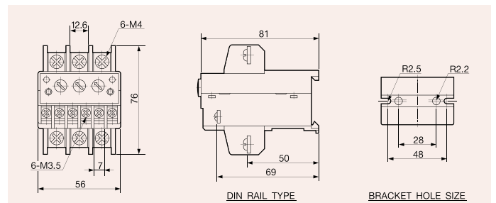
EOCR-DST / DS1T / DS2T / DS3T
