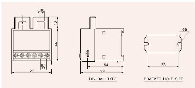
EOCR-SS1 / SS2
