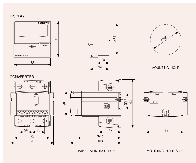
EOCR-PFZ
